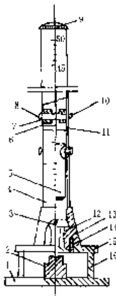
冲击试验器
