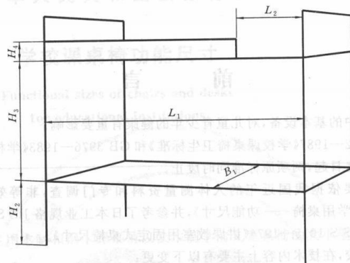
图3 双层床主要尺寸示意图
