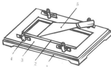
腻子刮涂器图
